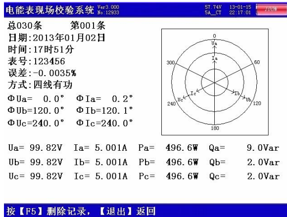
图十六、历史数据屏
