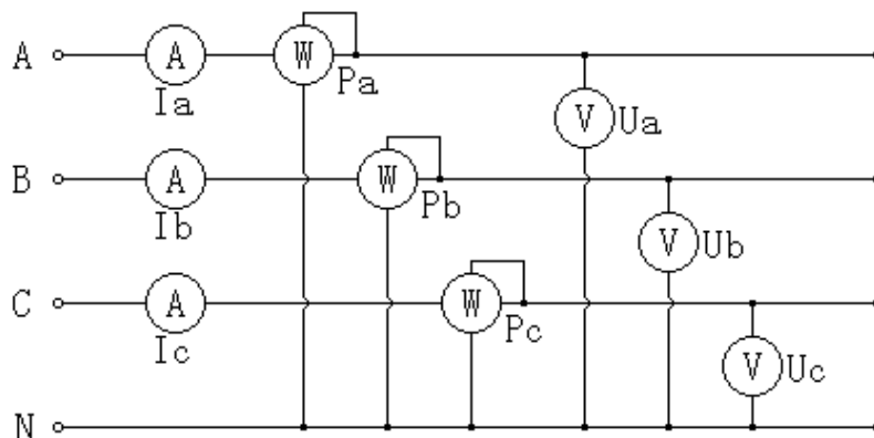
图十八、三相四线制测量原理图
