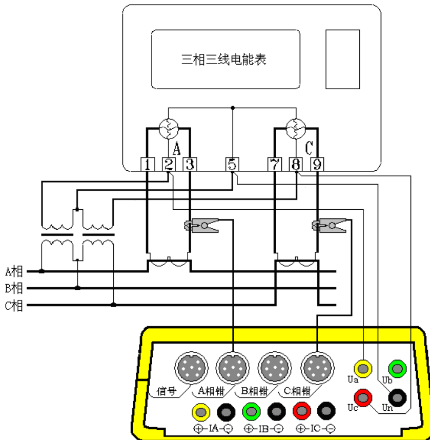
三相三线高压表计经钳表接入接线
