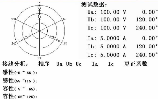
图九、矢量分析屏—三相四线
