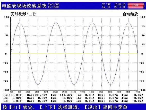
图十三、波形显示屏
