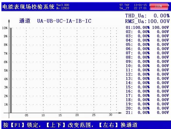
图十四、频谱分析屏
