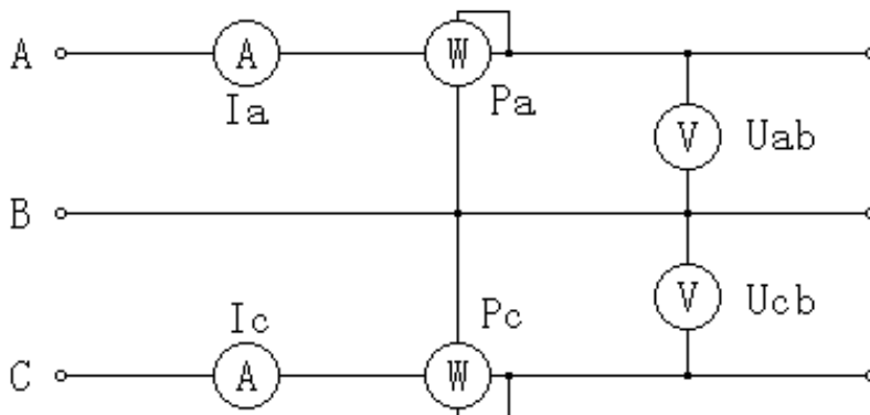
图十七、三相三线制测量原理图
