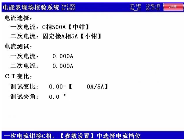
图十一、变比测试屏
