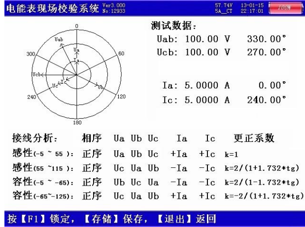
图十、矢量分析屏一三相三线
