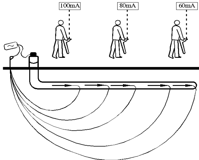
图 h 电流测量原理示意图
