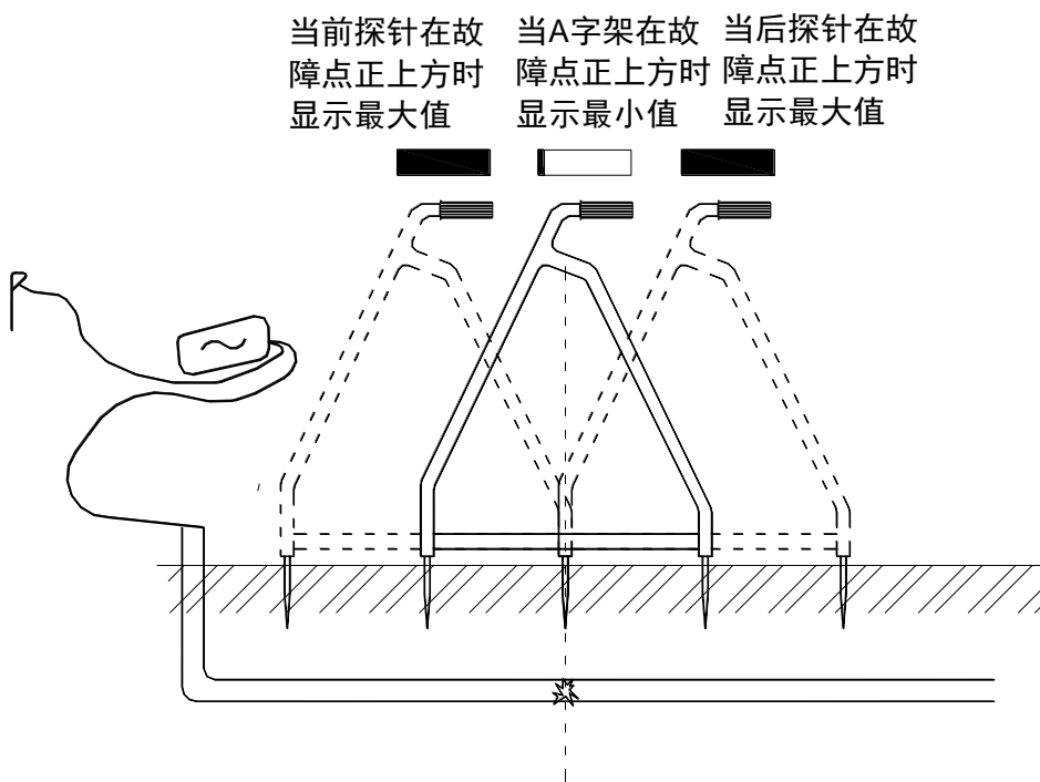
A 字架对管线故障点定位示意图
