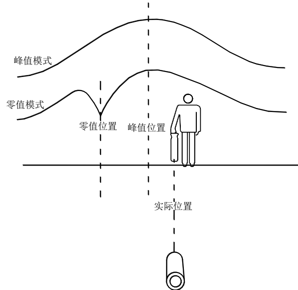
零值法和峰值法探测比较示意图
